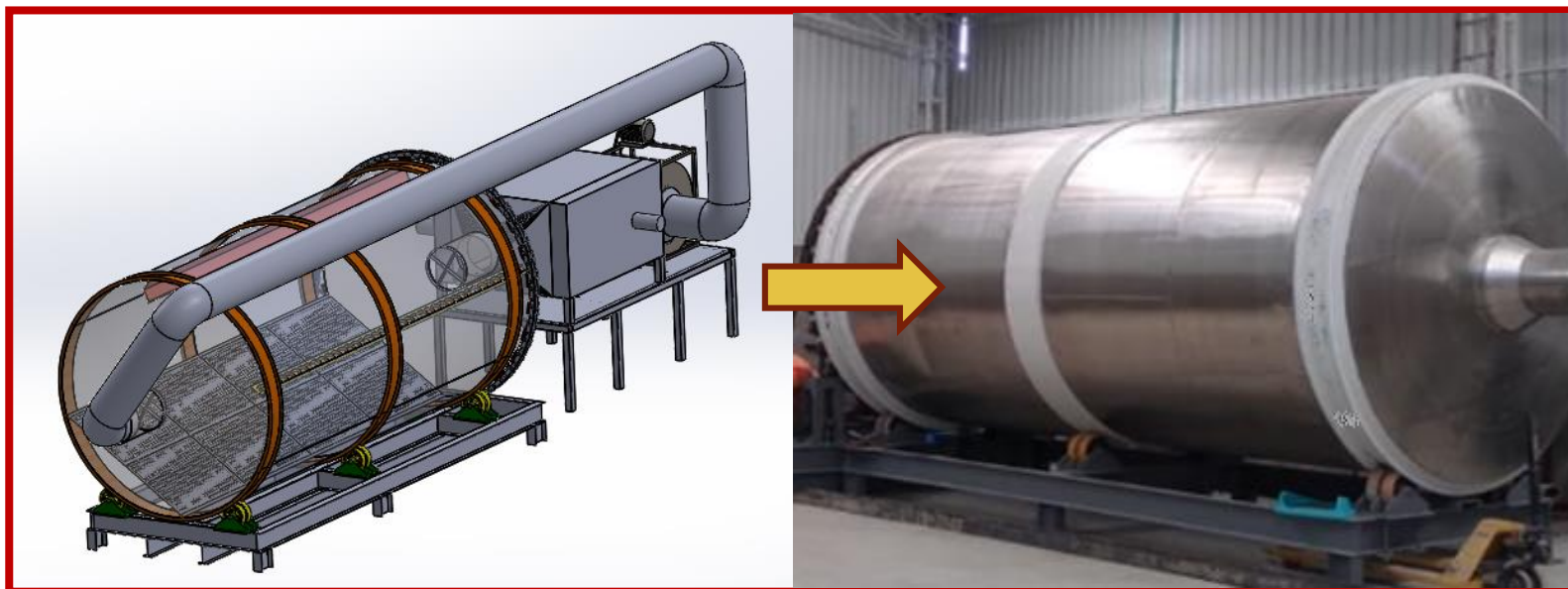
TANQUE ROTATIVO PARA PROCESO DE MALTEO Y SECADO/ INOX 304/25m3 LITROS PISO INTERNO ABATIBLE INOX 304
